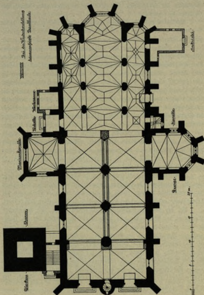
Grundriß der katholischen Pfarrkirche nach der Wiederherstellung, gezeichnet von Regierungsbaumeister Stiehl.
