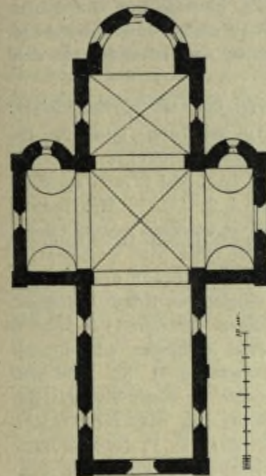
Mutmaßlicher Grundriß der ältesten kirchlichen Anlage Münsterbergs, gezeichnet von Regierungsbaumeister Stiehl.
