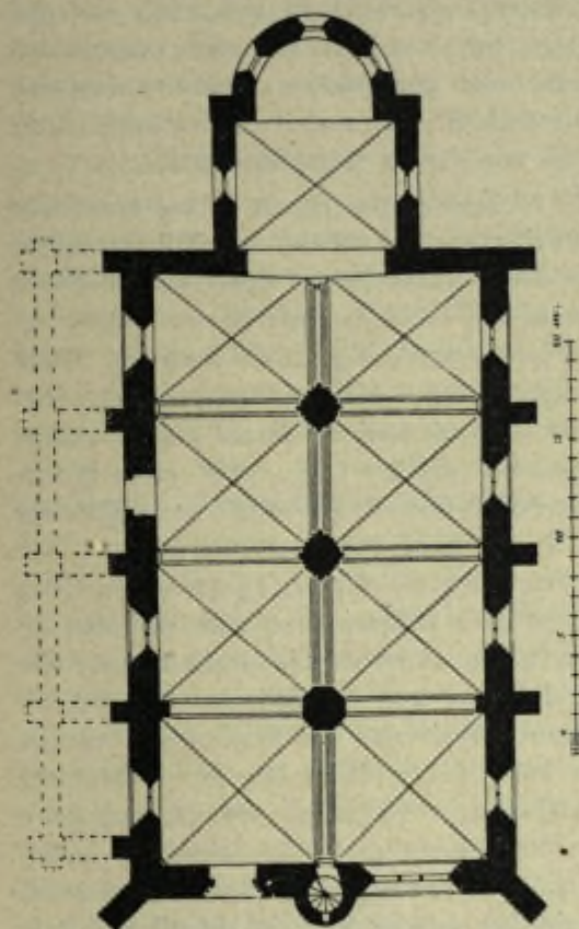
Ursprünglicher Langhausbau der kath. Pfarrkirche, gezeichnet von Regierungsbaumeister Stiehl.
