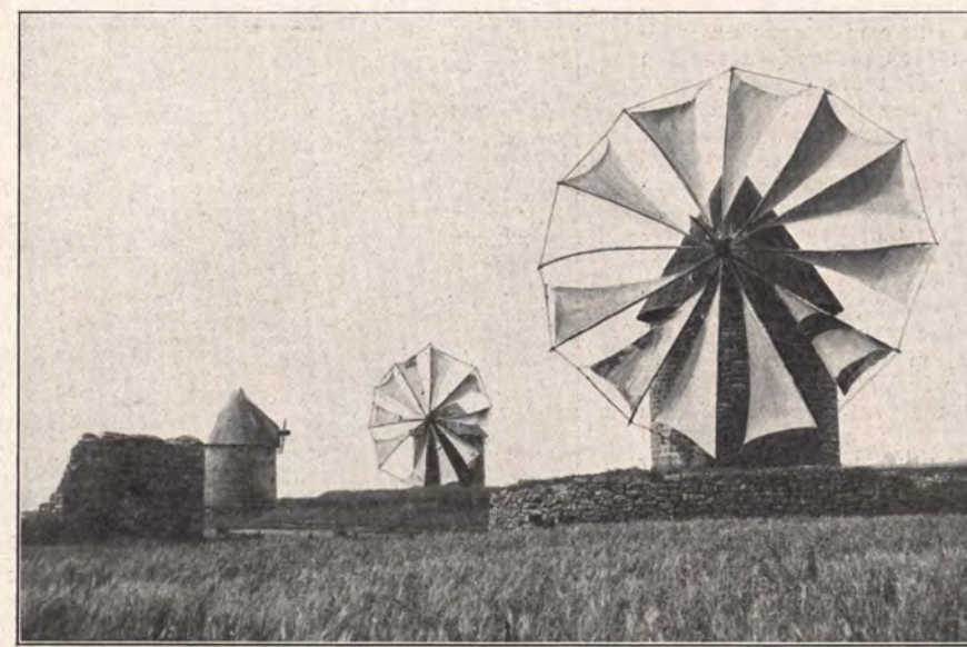
Mazedonische Windsegelmöhlen.
