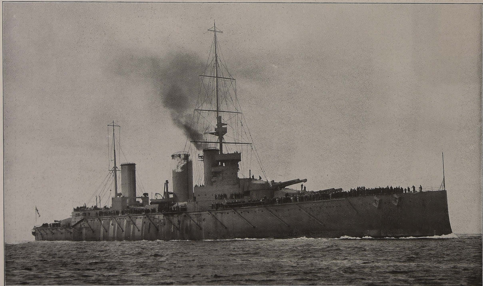
Schlachtkreuzer „Queen Mary“. (Wasserverdrängung: 30 000 t; Artillerie: Acht 34,3-cm- und sechzehn 10,2-cm-Geschütze; Besatzung: 1020 Mann.)
