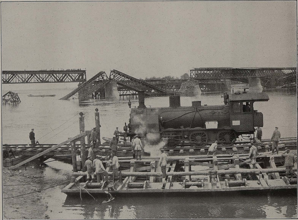
Auf der Weichsel bei Warschau: Überführung einer Lokomotive von einem Ufer zum andern auf einem Floße durch deutsche Eisenbahntuppen. (Phot. A. Semede.)
