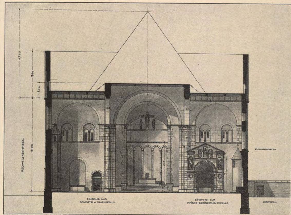
QUERSCHNITT GEGEN DEN CHOR DER KRIEGSGEDÄCHTNISKIRCHE IN NÜRNBERG UND PORTAL ZUR KAPELLE Text unten u. S. 47
