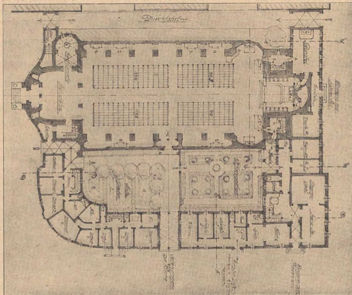
Karl Hocheder (München) Grundriss des Erdgeschosses der Kirche, des Pfarrhauses und der Mesnerwohnungen, mit Gärten. Links dahinter der Prozessionshof
