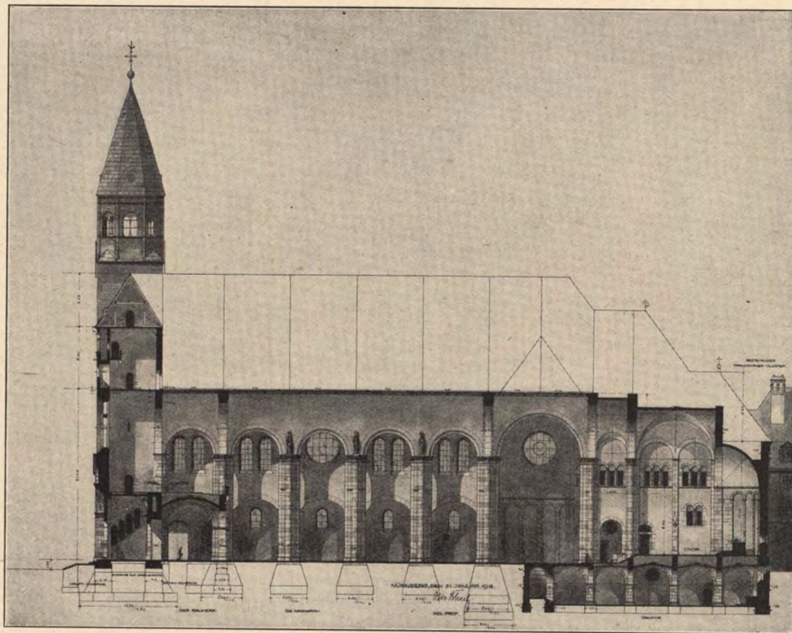
LÄNGENSCHNITT DER KRIEGSGEDÄCHTNISKIRCHE IN NÜRNBERG. — Vgl. Text S. 43
