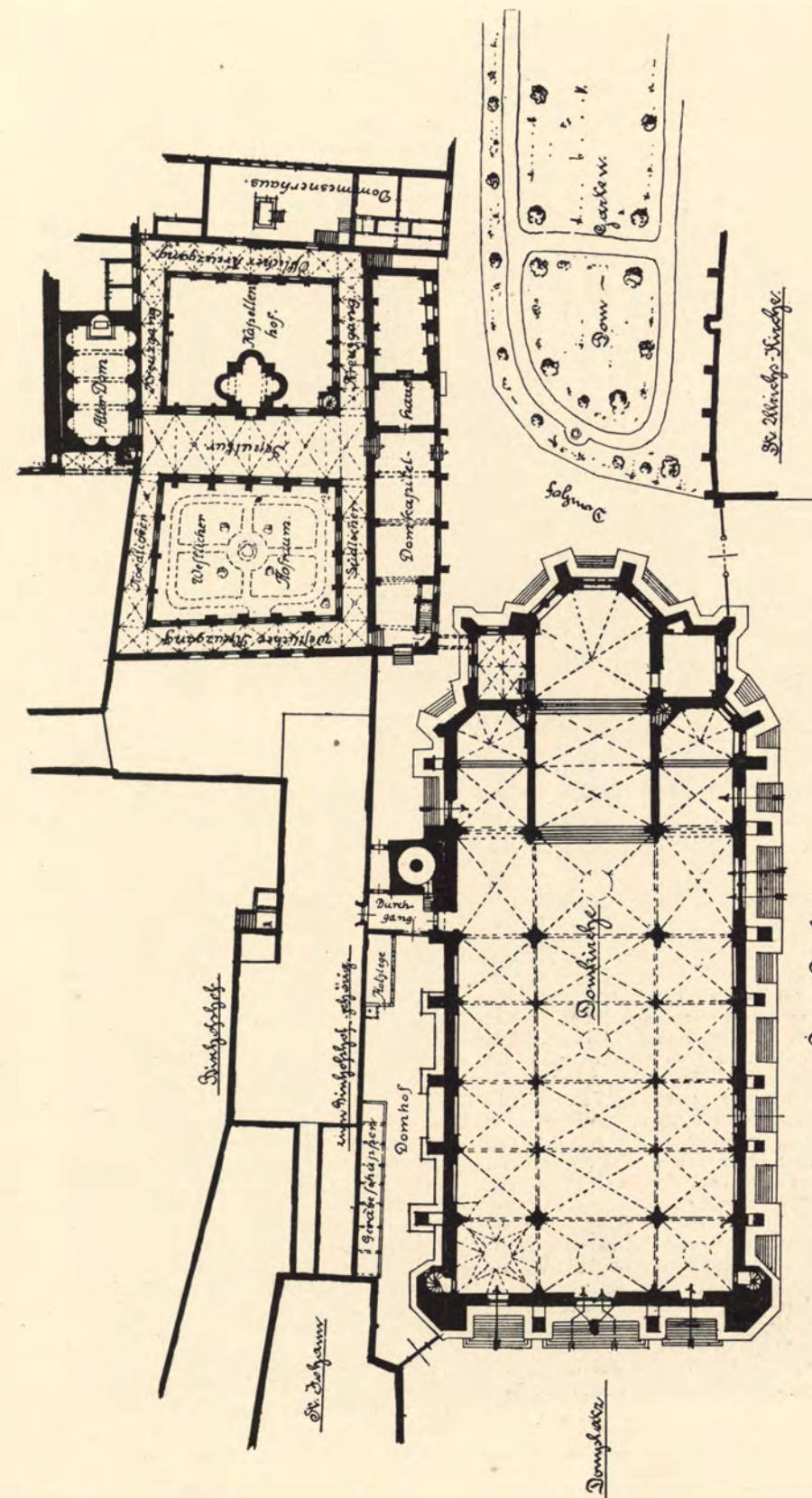
LAGEPLAN DES DOMES IN REGENSBURG Text S. 234. — Vgl. S. 128
