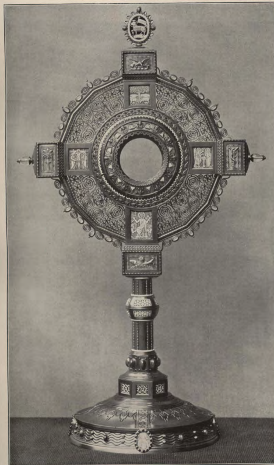
JOHANN VORFELD (KEVELAER) MONSTRANZ Silber vergoldet. Entwurf von Maler Brey, Geldern. — Deutsche Werkbundaussstellung Köln 1914
