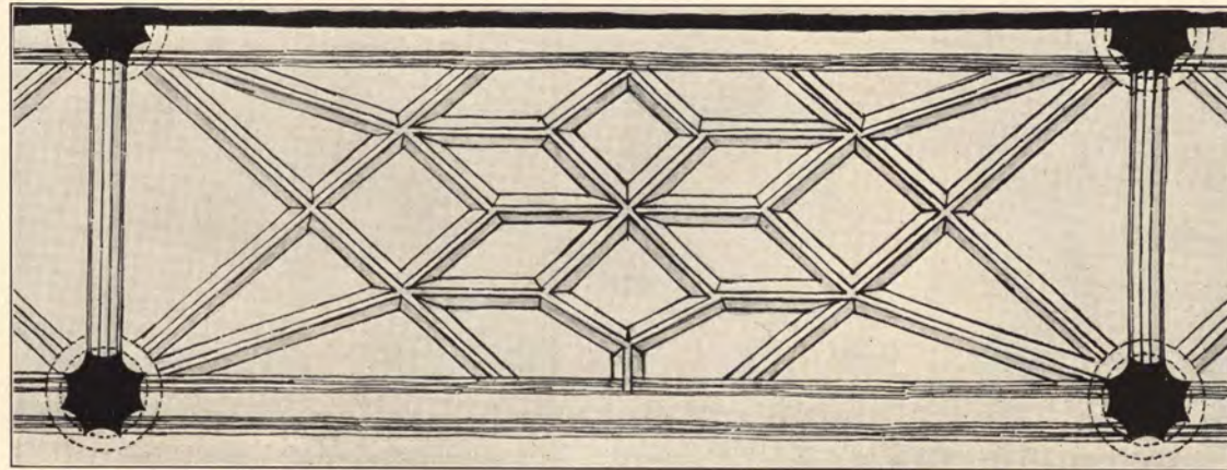
WÖLBUNG DER EMPORE IN DER MARIENKIRCHE ZU HALLE a. d. S. Zeichnung von Hugo Steffen
