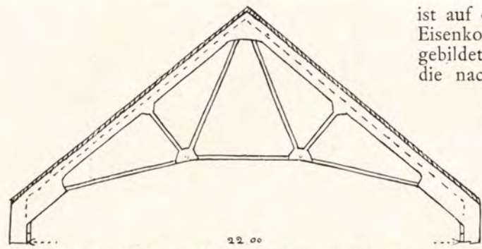
DIAGONALDACHBINDER DER GARNISONSKIRCHE IN KIEL, VON WEIRICH UND REINKEN Vgl. Abb. S. 365. Text S. 365
