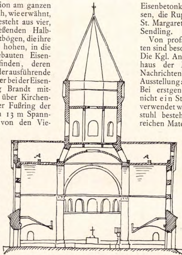
SCHNITT DER KREUZKIRCHE IN DÜSSELDORF VON SCHLEICHER Text nebenan
