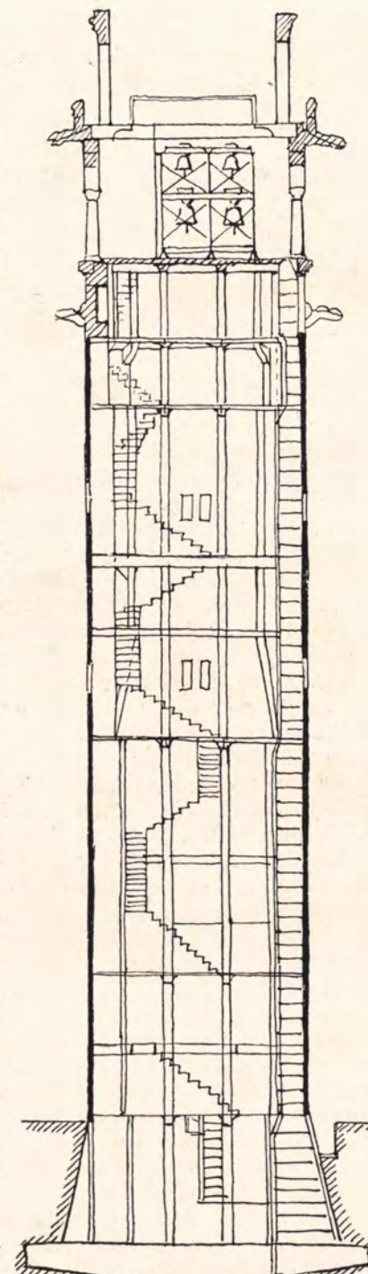
TURMSCHNITT DER NEUEN MARKSKIRCHE IN STUTTGART, VON OBERBAURAT DOLMETSCH Text nebenan u. S. 364
