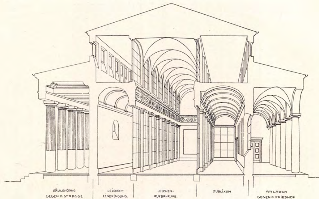
Perspektivischer Schnitt durch die Leichenhallen des östlichen Friedhofes in München Text S. 270
