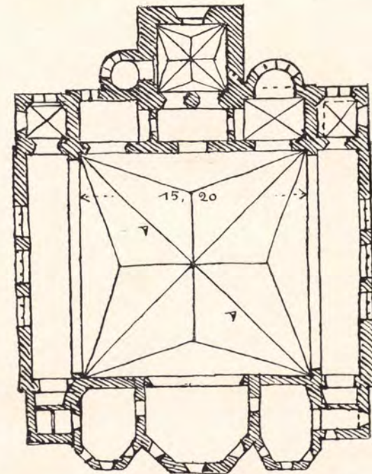
GRUNDRISS DER KATH. GARNISONSKIRCHE IN KIEL, ENTWORFEN VON KELM Text nebenan
