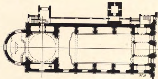
GRUNDRISS DER KLOSTERKIRCHE ZU DIessen Text S. 342
