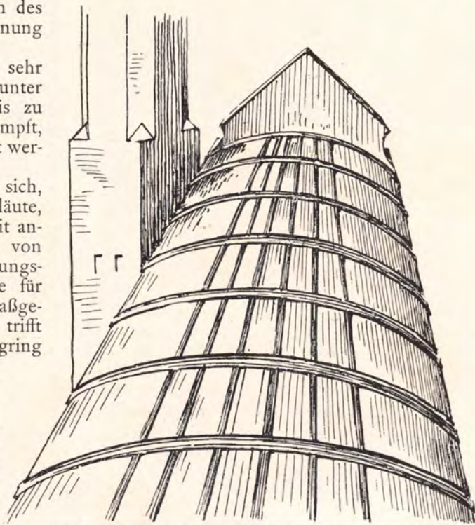
EISENBETONGEWÖLBE DER MARKUSKIRCHE IN STUTTGART Von oben gesehen. Text S. 363 und nebenan
