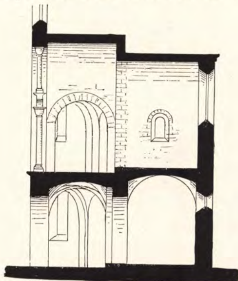
Fig. 18. Ottmarsheim, Schnitt durch den Chor
