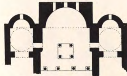
Fig. 8. Chor der Nikolauskirche zu Myra
