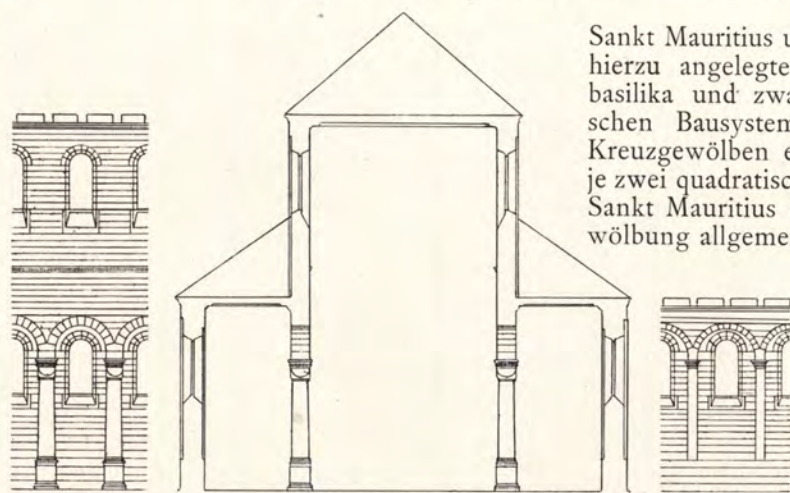
Längenschnitt und Querschnitt des Langhauses — Längenschnitt der Abseiten der ursprünglich flach gedeckten Säulenbasilika in Maria Laach
