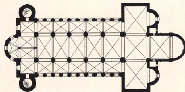
Grundriß der im Anfang des 13. Jahrhundert vollendeten gewölbten Pfeilerbasilika mit zwei Chören der Benediktiner-Abtei Maria Laach Text oben
