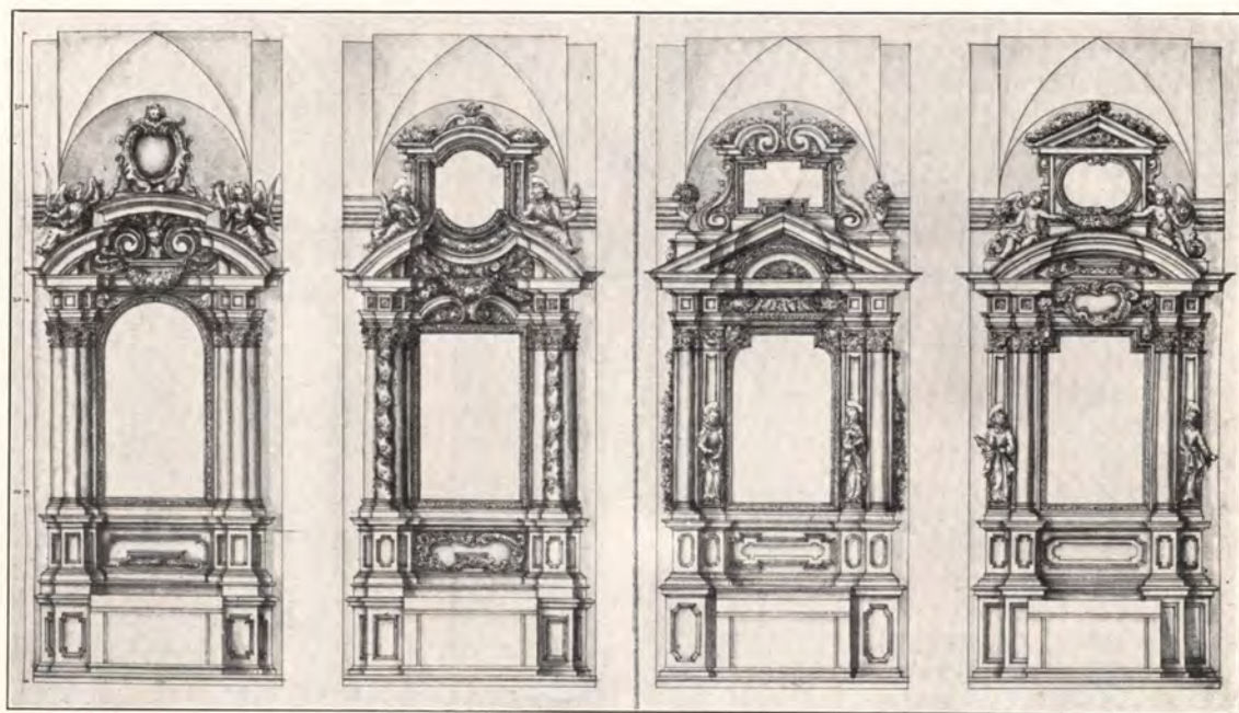
ENTWÜRFE ZU DEN SEITENALTÄREN IN DER ABTEIKIRCHE WALDSASSEN (1688) Text S. 54
