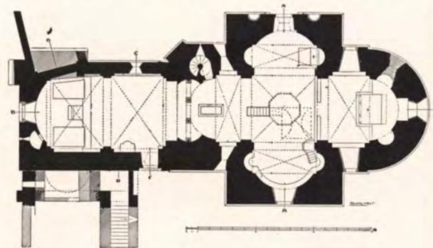
GRUNDRISSE DER UNTERKIRCHE ZU SCHWARZ-RHEINDORF Mit Genehmigung des Provinzialkonservators der Rheinprovinz
