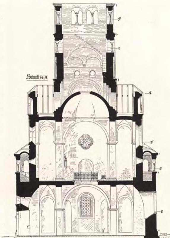
QUERSCHNITT DER KIRCHE IN SCHWARZ-RHEINDORF Mit Genehmigung des Provinzialkonservators der Rheinprovinz
