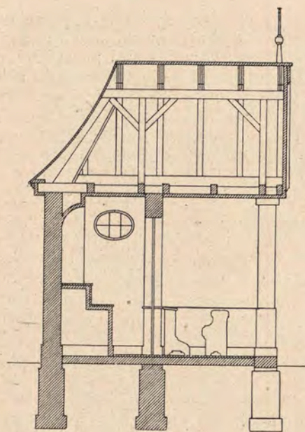
Hans Grüssel Kapelle, Längenschnitt
