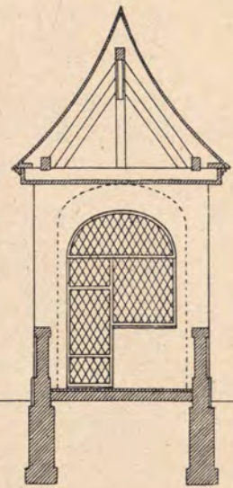
H. Grüssel Kapelle, Querschnitt
