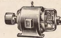
(Kompensierter Drehstrommotor) Synasyn-Motor D. R. P. \cos \varphi = 1 oder voreilend Einziger seit drei Jahren bewährter Motor ohne Blindverbrauch
