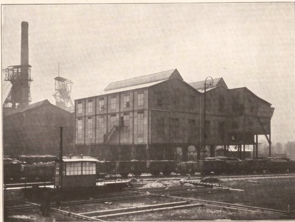
Bild 1 Separation und Schiebebühne Ludwigsglückgrube b. Vorfigwerk
