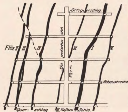
Fig. 3. Stapelschacht (Saigerriess)
