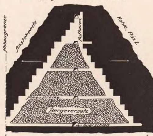
Abbau im Flöz selbst. Fig. 4. (folgt der Ebene von Flöz I).
