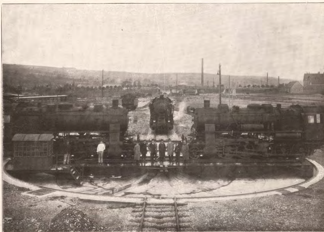
Bild 3 Lokomotiv-Drehscheibe, 23 m Durchmesser, 240 t Tragkraft
