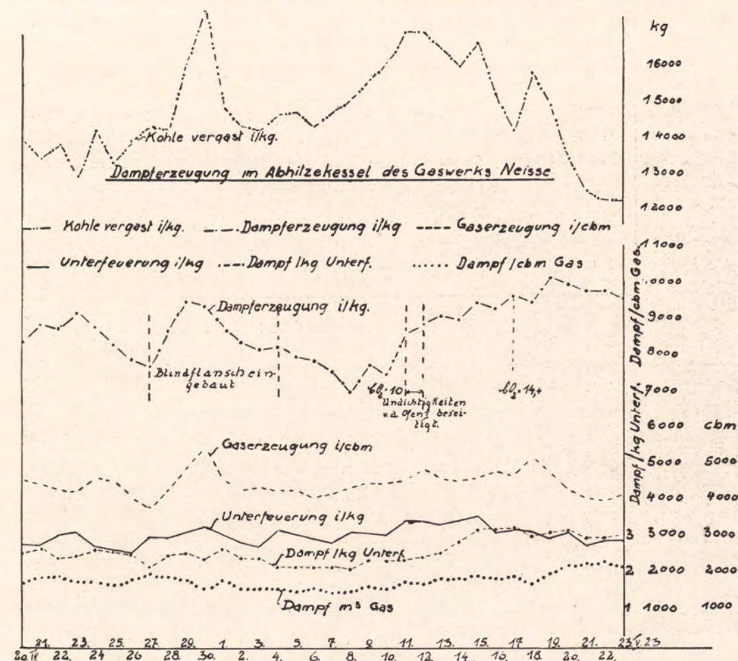
Dampferzeugung im Abhizekessel des Gaswerkes Neisse.
