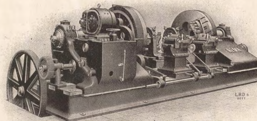
Lokomotiv-Radsatz-Drehbank „LRD“
