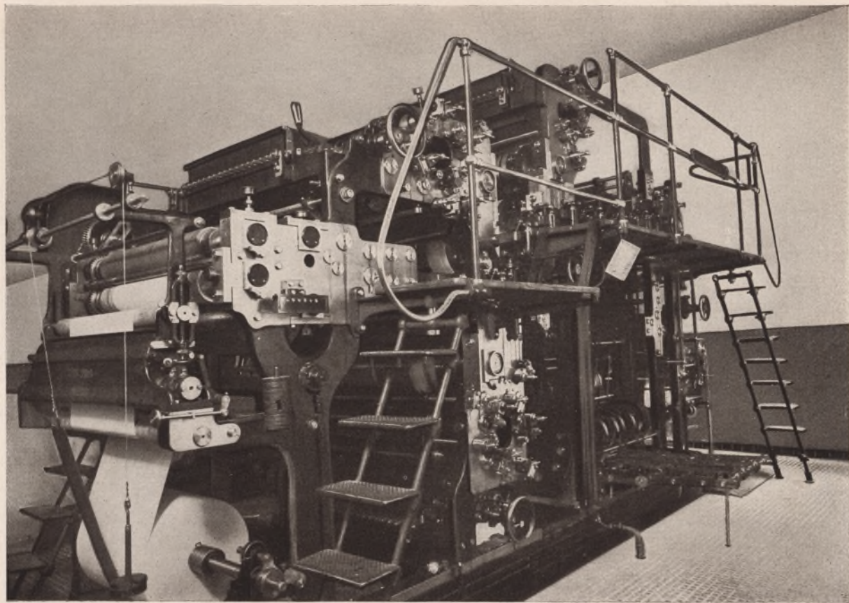
Variable Rotationsmaschine
