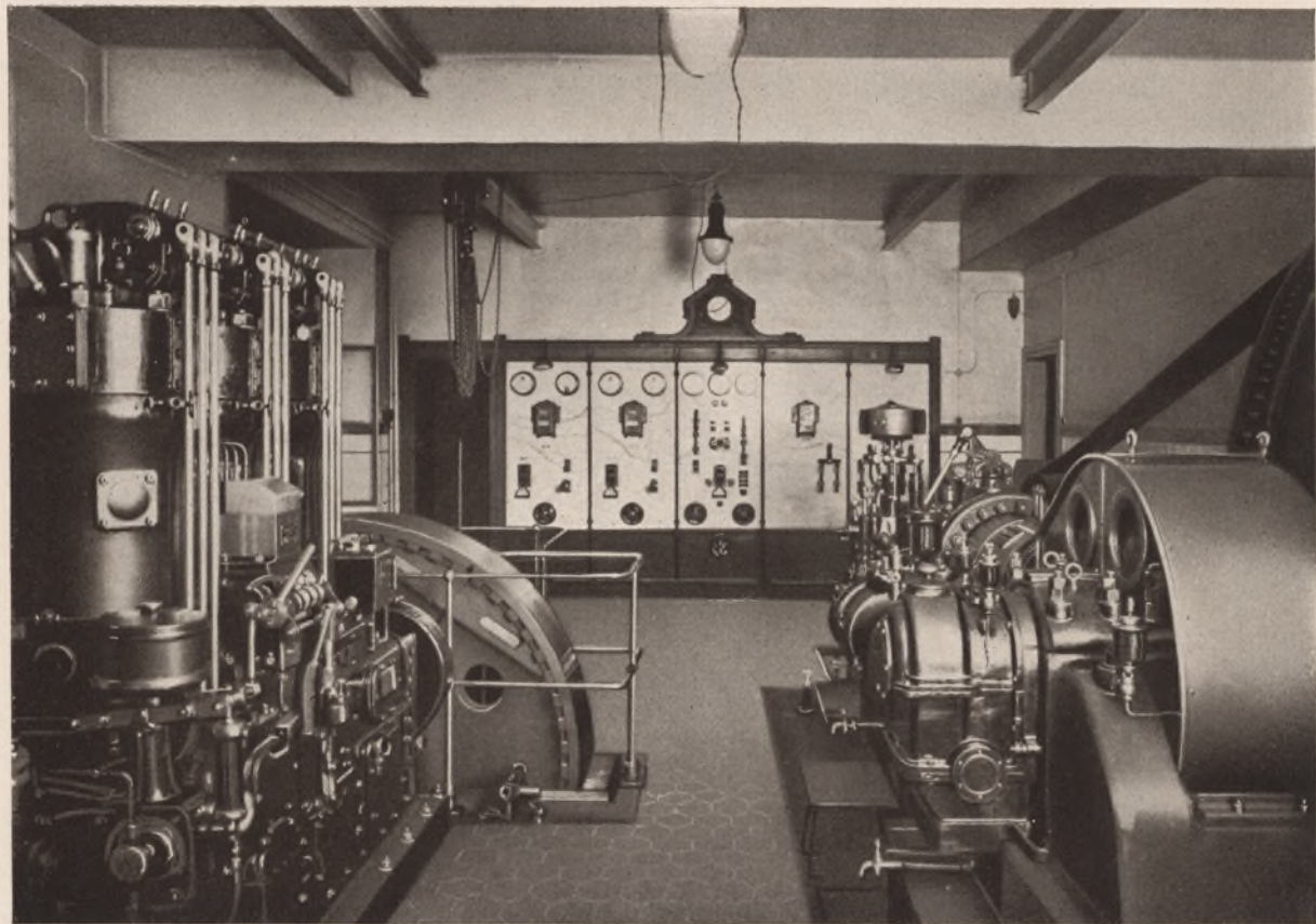
Dieselmotoren-Kraftanlage
