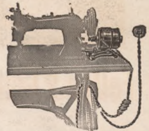
Universal-D. R. G. M.-Näh- maschinenmotor m. Kugel- lagerung, Fussregler usw. Ohne Montage sof. betriebsbereit. Für angestrengten gewerblichen Dauerbetrieb; verbraucht in etwa 66 Betriebsstunden nur 1 Kw-Std. annähernd 1/12 P. S.-Leistung Man verlange Anerkennungs- schreiben!
