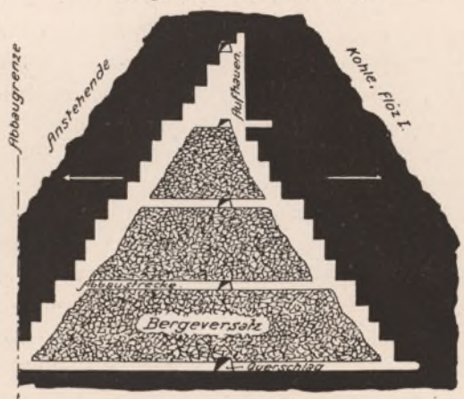
Abbau im Flöz selbst. Fig.4. (folgt der Ebene von Flöz I).
