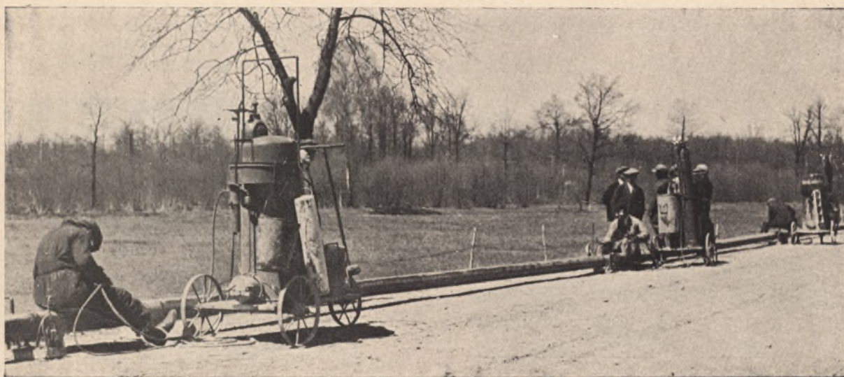
Widok spawania gazociągu Daszawa-Lwów
