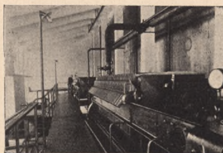
Prasy filtracyjne
