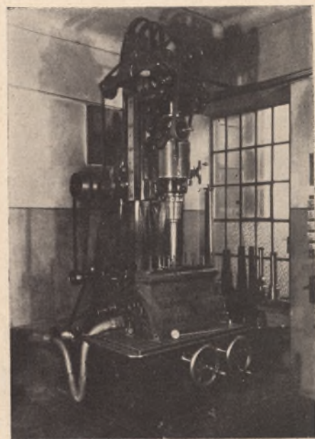
Szlifierka cylindrów samochodowych.
