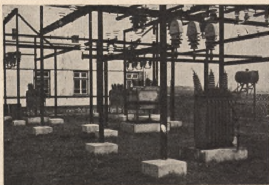
Stacja powietrzna transformatorowa w Lubieniu Wielkim 30/6 KV 50 KVA
