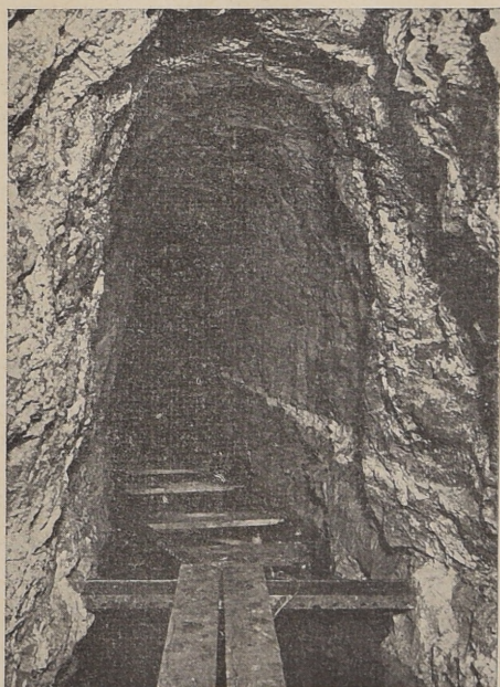
Sztolnia żeglowna wykuta w dolomicie, zabarwionym kolorowo skamieniałymi ściekami. — Łódź, gotowa do jazdy w sztolnię.
