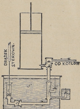
Szosta maszyna parowa, zbudowana na Górnym Śląsku w Ozimku i puszczona w ruch 1798 r. w rewirze suchogórskim pod Tarnowskimi Górami
