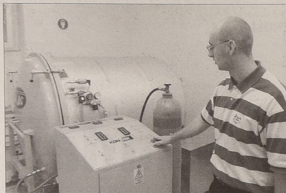
Tomasz Cygan obsługuje urządzenie do dezynfekcji i suszenia książek.
