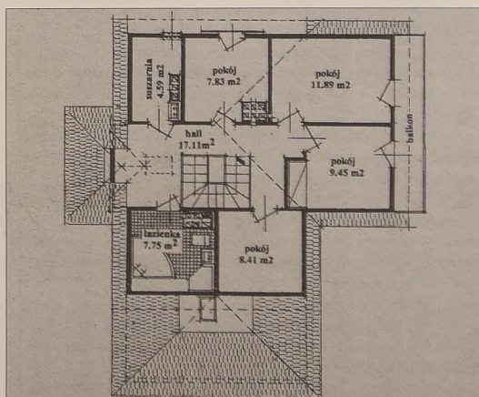
Rzut użytkowego poddasza.
