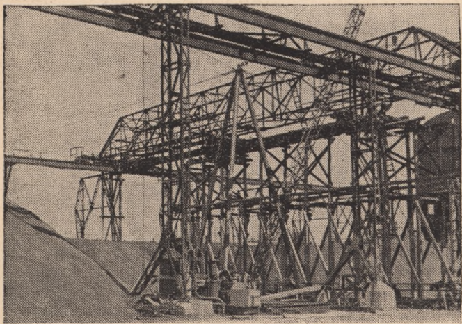
ELEKTROWNIA GŁÓWNA WE WROCŁAWIU Przesuwnica węglowa w maju 1946 r.
