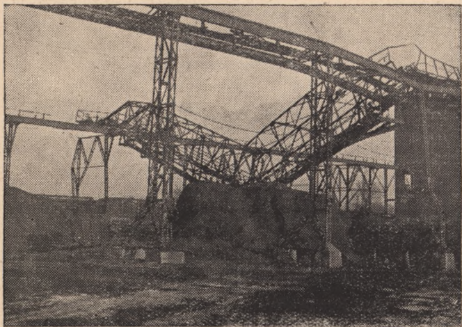
ELEKTROWNIA GŁÓWNA WE WROCŁAWIU Przesuwnica węglowa w maju 1945 r.
