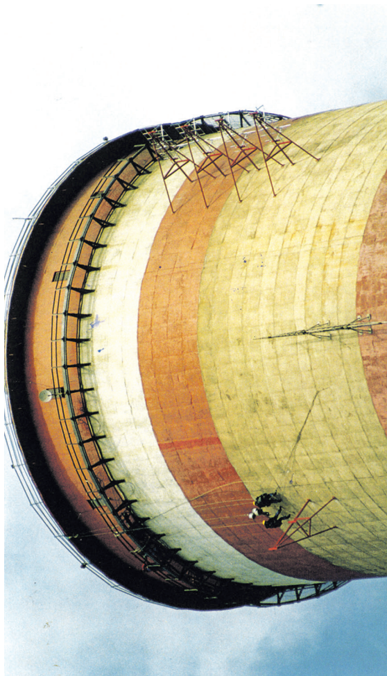
Montaż anten rozgłośni diecezjalnej na płaszczu komina Elektrowni „Opole” w Brzezinie na wysokości ok. 100 m, w lecie 1997 r.
